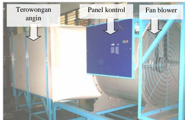
Gambar 6. Terowongan angin yang digunakan dalam penyelidikan unjuk kerja model-model kincir angin.
