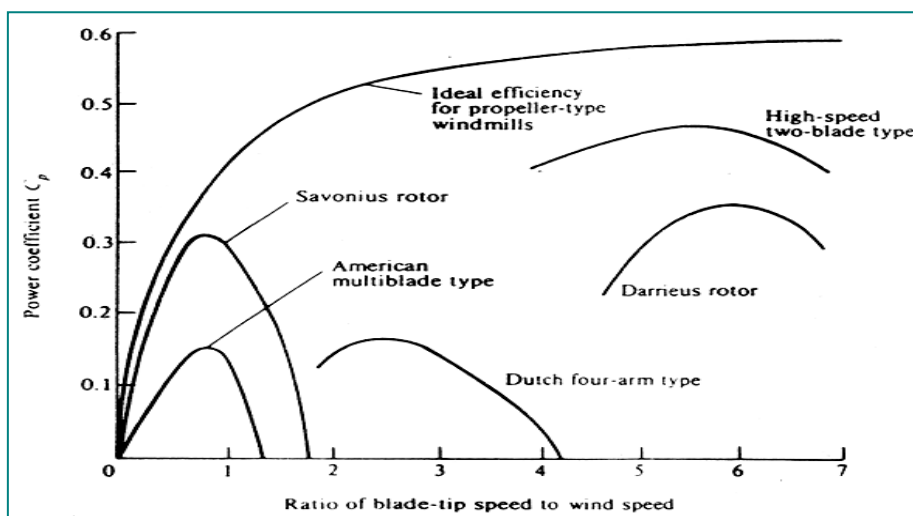
Gambar 2. Kurva hubungan koefisien daya, C_p , dan tip speed ratio , tsr , untuk berbagai tipe kincir angin standard [1].
