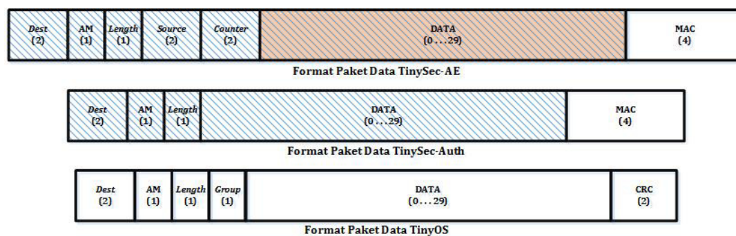
Gambar 5. Format Paket Data TinySec dan TinyOS. Ukuran Byte setiap Field Ditunjukkan di Bawah Label. Field yang Diarsir Menunjukkan bahwa Field tersebut Terlindungi dengan Adanya MAC. Pada TinySec-AE, Field Datanya Terenkripsi.
