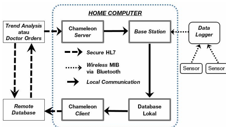
Gambar 2. Blok Diagram HIS untuk Home Monitoring
