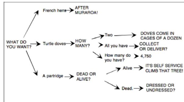
Gambar 2. Pohon percakapan
