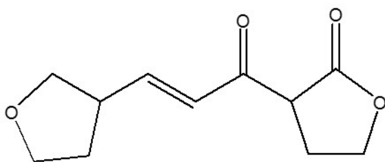
Gambar 2. Struktur laktogenin
