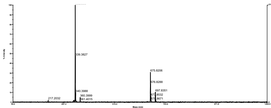
Gambar 2. Spektra massa dari senyawa hasil sintesis
