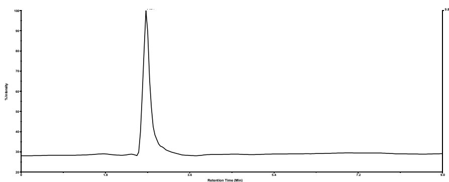
Gambar 1. Kromatogram LC senyawa hasil sintesis
