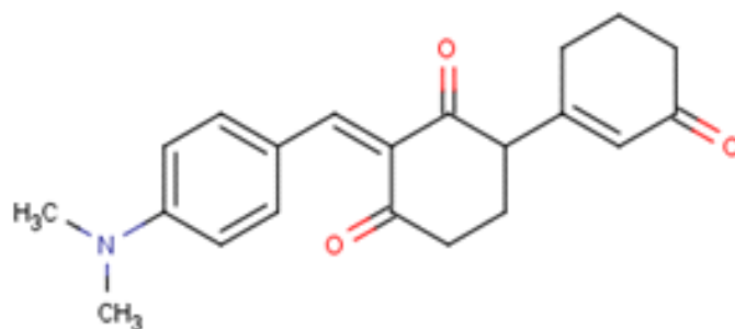
Gambar 5. Struktur senyawa 2-(4-(dimetilamino)benzilidena)-4-(3-oksosiklohex-1-enil) sikloheksana-1,3-dion
