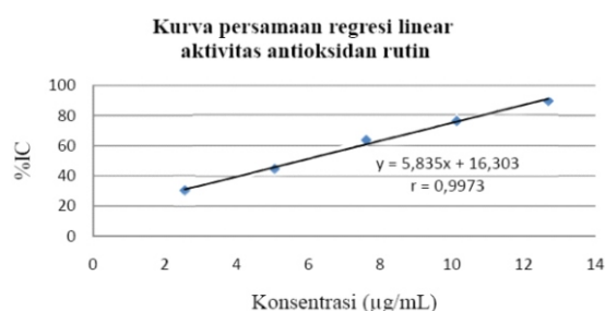
Gambar 5. Kurva persamaan regresi linier aktivitas antioksidan rutin
