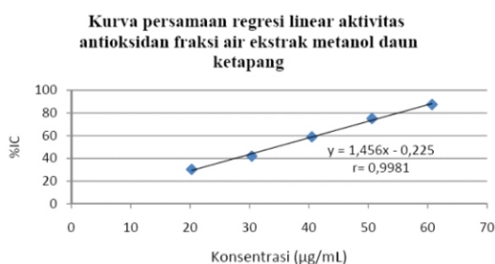
Gambar 6. Kurva persamaan regresi linier aktivitas antioksidan fraksi air ekstrak metanolik daun ketapang
