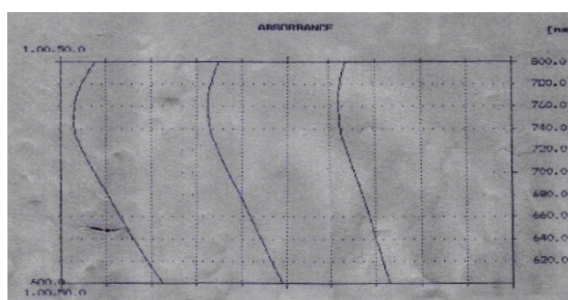
Gambar 4. Penetapan \lambda_{\text{maks}} asam galat dalam tiga seri kadar ditambah pereaksi Folin- Ciocalteu
