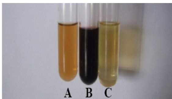
Gambar 1. Hasil uji pendahuluan aktivitas antioksidan: A) Larutan DPPH ditambah fraksi air ekstrak metanolik daun ketapang; B) Larutan DPPH (kontrol negatif); dan C) Larutan DPPH ditambah larutan rutin (kontrol positif)
