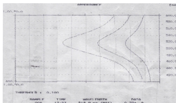
Gambar 3. Spektra UV \lambda_{\text{maks}} DPPH pada tiga seri konsentrasi
