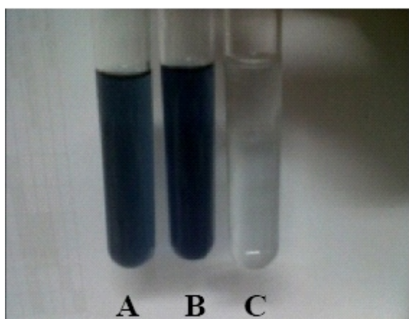
Gambar 2. Hasil uji pendahuluan fenolik total: A) Pereaksi Folin Ciocalteu ditambah fraksi air ekstrak metanolik daun ketapang; B) Pereaksi Folin Ciocalteu ditambah asam galat; dan C) Larutan blanko
