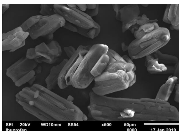
ibuprofen
