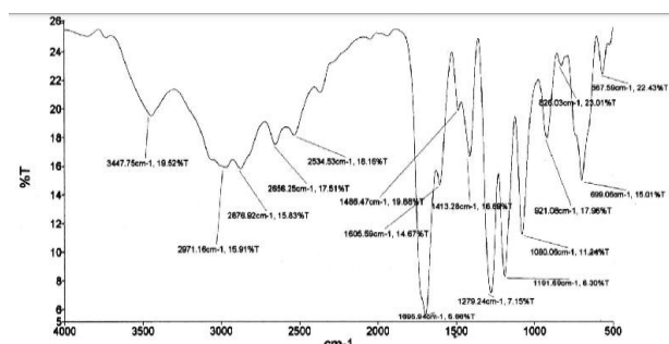
Gambar 2. Spektrum inframerah senyawa asam 2-(3-(klorometil) benzoiloksi)benzoat
