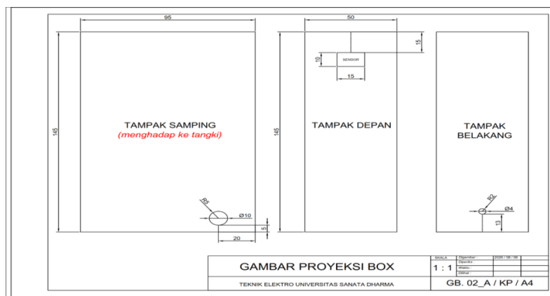
Gambar 4. Rancangan Proyeksi Box dengan AutoCAD
